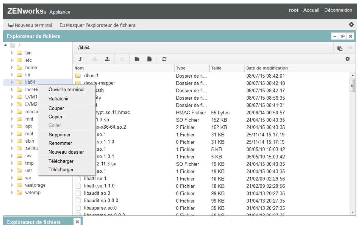
Figure 6-5 Explorateur de fichiers
