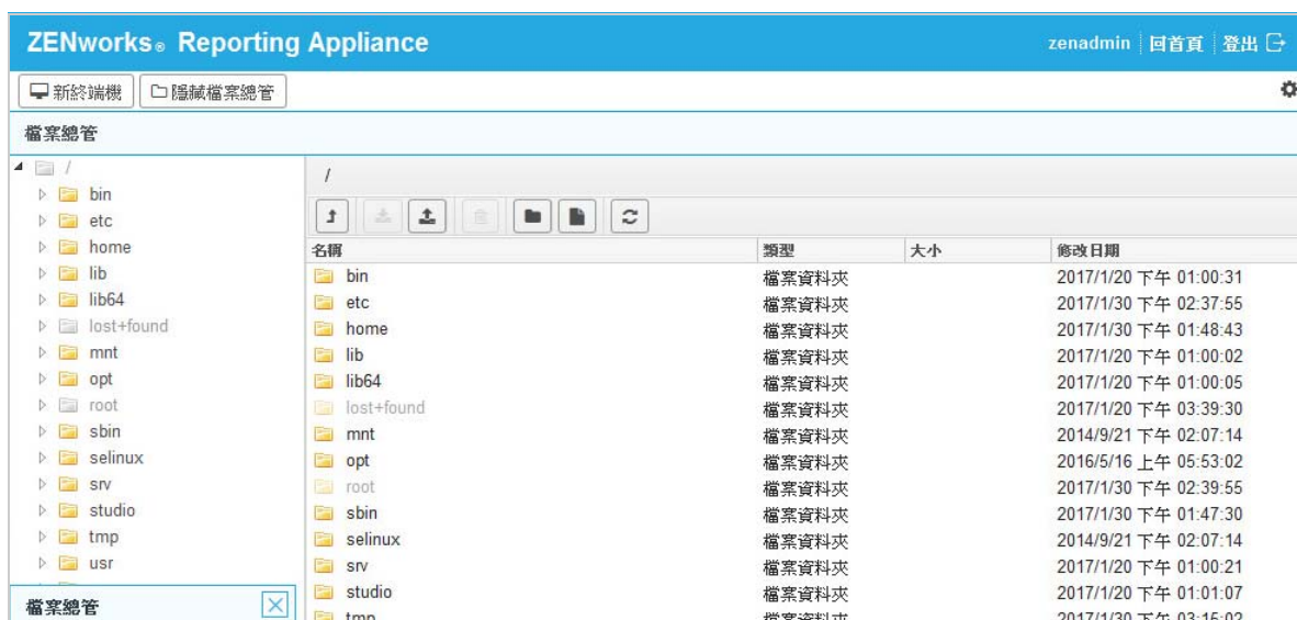
圖 6-5 檔案總管
