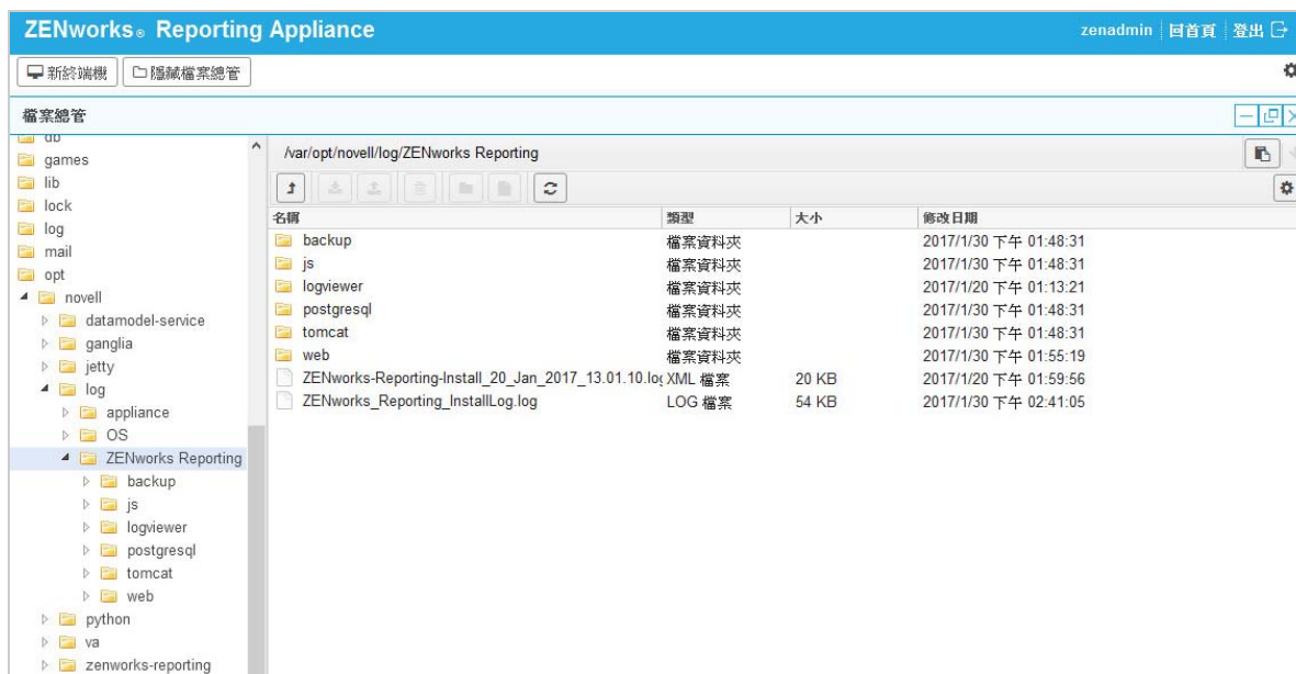
圖 6-6 記錄
