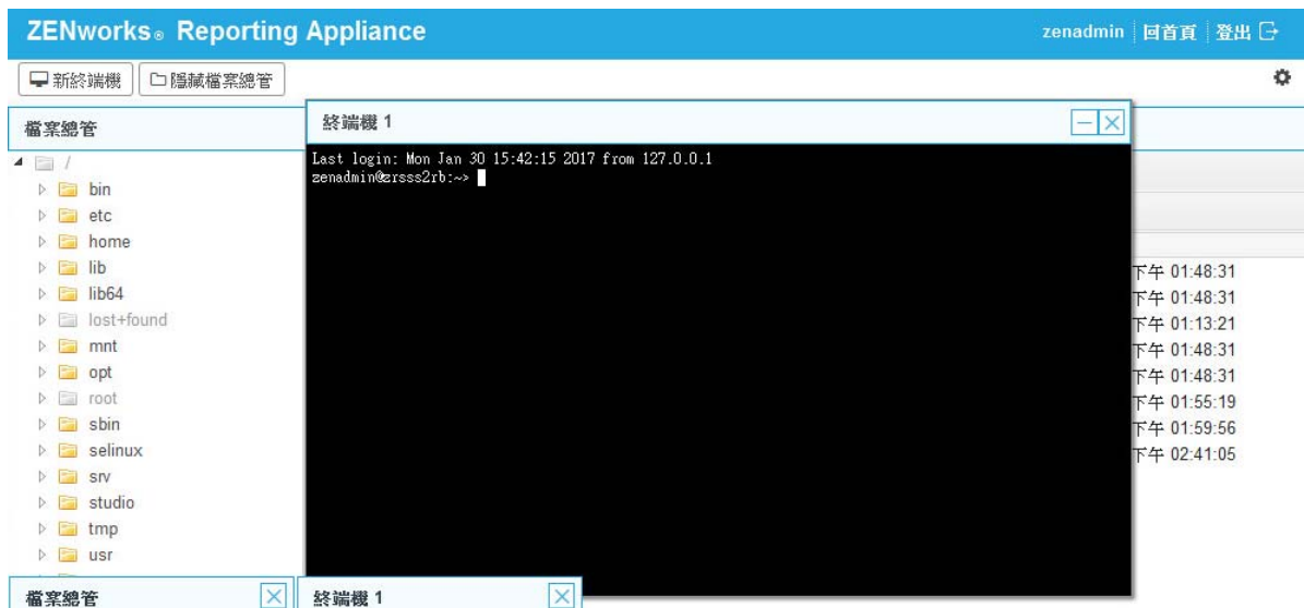
圖 6-4 終端機
